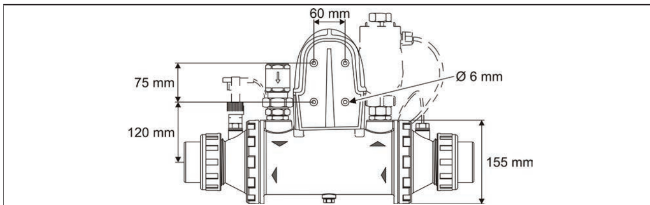
Abmessungen für die Befestigung Heat Line + und Heat Line SC
