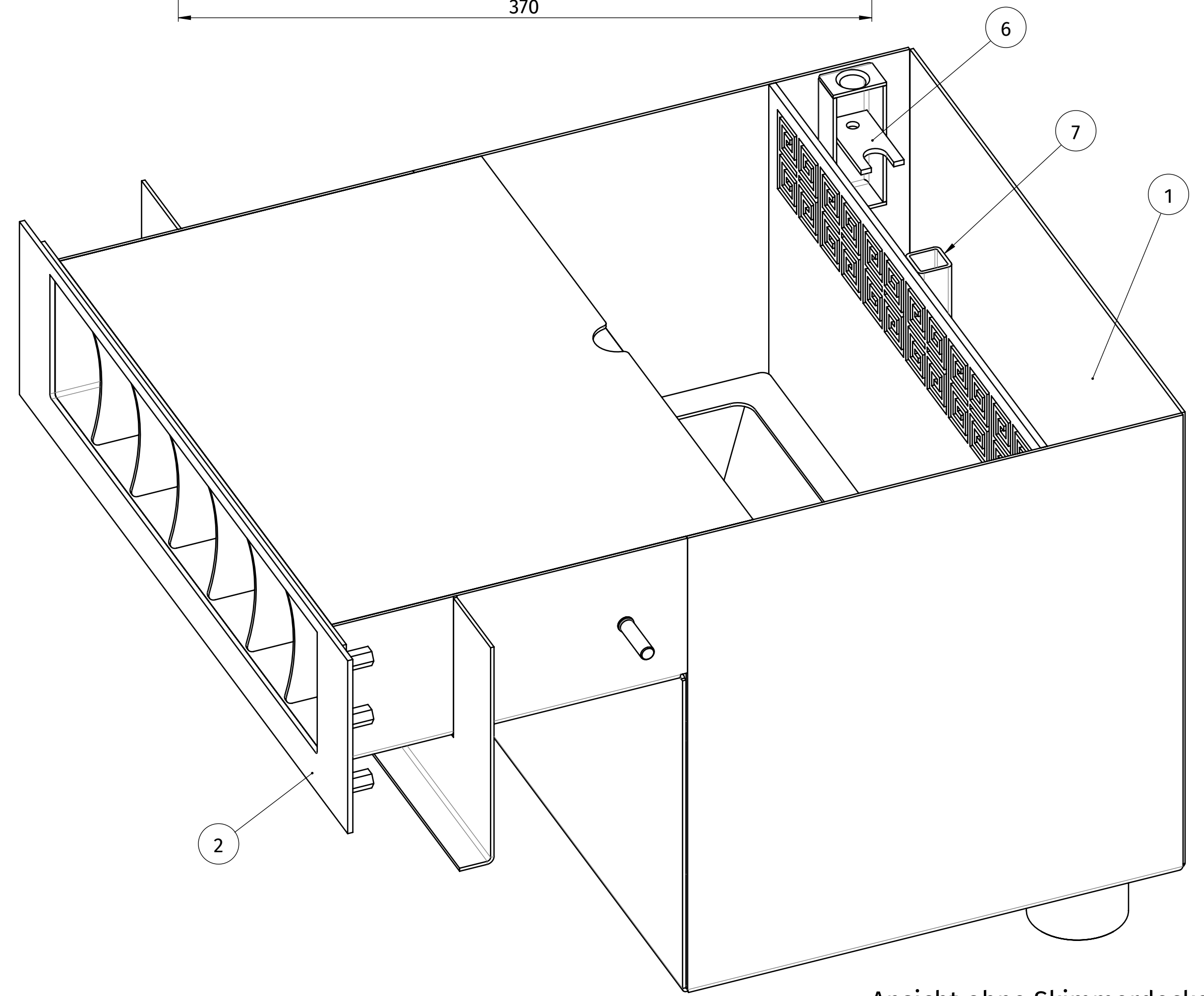
Ansicht ohne Skimmerdeckel
