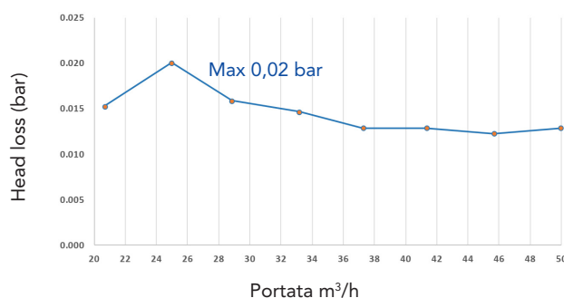
Perdita di pressione (bar) - DN 80
