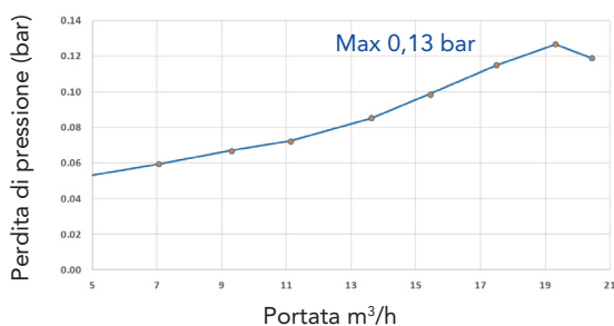
Perdita di pressione (bar) - DN 40
