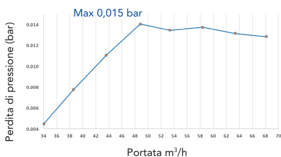
Perdita di pressione (bar) - DN 100
