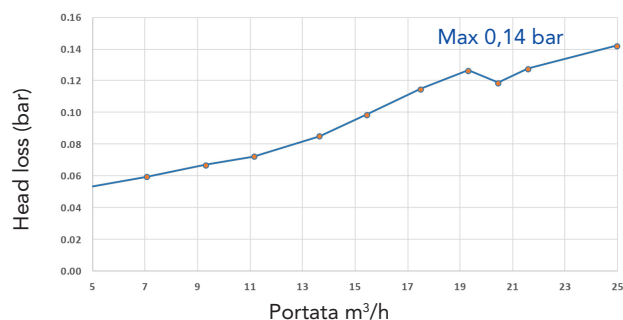
Perdita di pressione (bar) - DN 50
