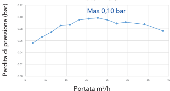
Perdita di pressione (bar) - DN 65
