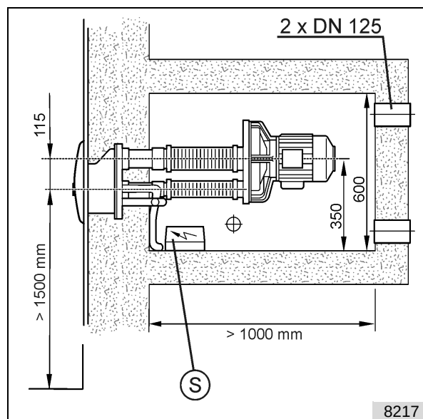
fig. 10: Vue de dessus de la cuve de la pompe
