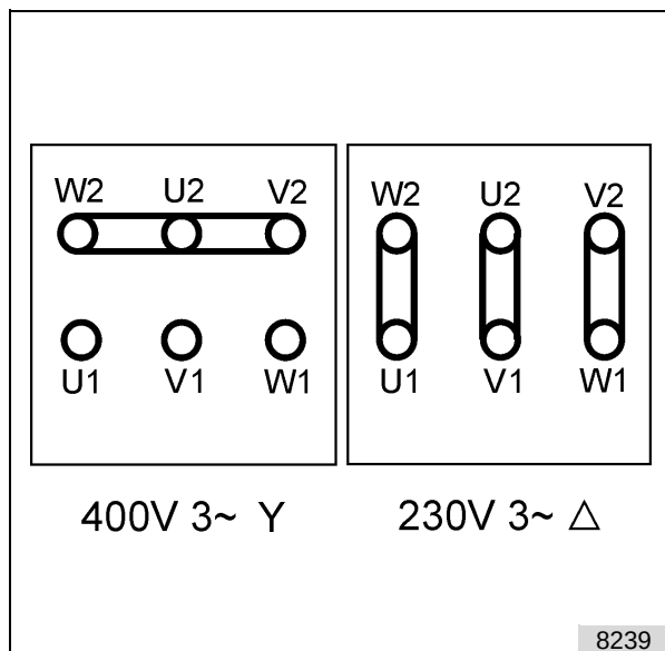
fig. 32: Schéma de principe pour courant triphasé 400/230 V
