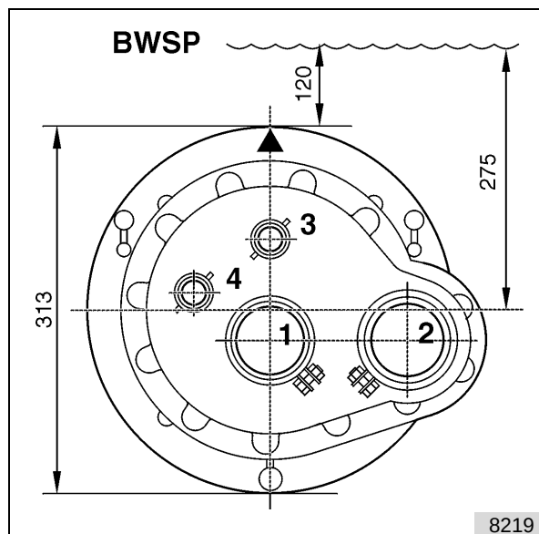
fig. 12: Vue de dos de la pièce à sceller
