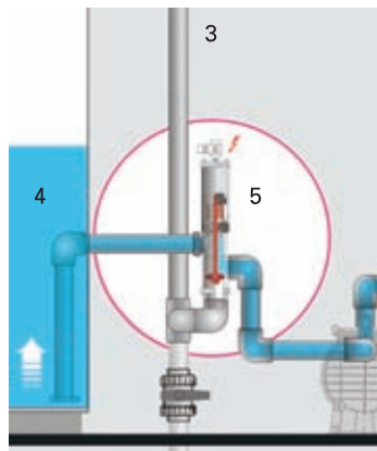
Modalità canale a sfioro
