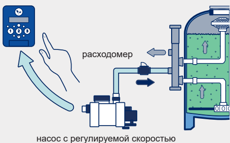
насос с регулируемой скоростью
