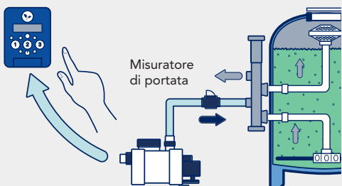
Pompa a velocità variabile
